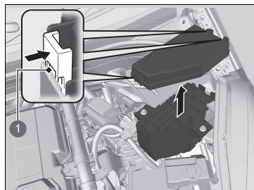
1 Výčnělky
