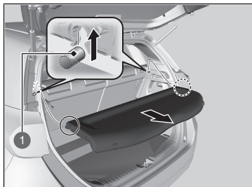
1 Podpěrná tyč
